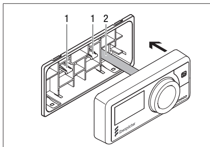
1 Защелки
